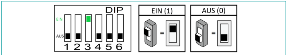
DIP-Schalter OBEN = EIN | DIP-Schalter UNTEN = AUS
